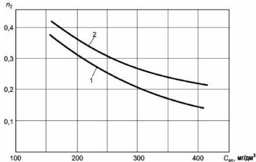
Рисунок В.1 - Залежність показника ступеня n_2 від концентрації завислих речовин C_{оп} у міських стічних водах при ефекті освітлення 50 % та 60 %
